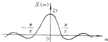
图 1-7 矩形脉冲的频谱
