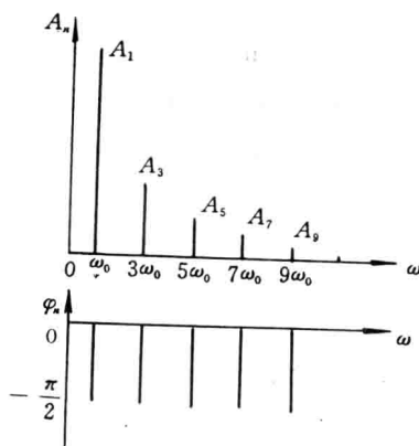
图 1-3 周期性方波频谱图
