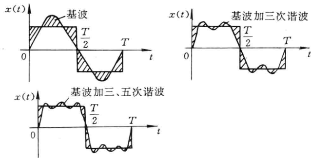
图 1-4 谐波项数与方波近似程度
