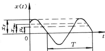
图 1-5 周期信号的强度
