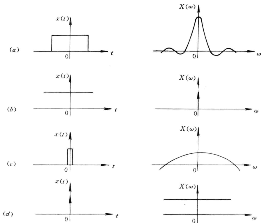
图 1-8 脉冲宽度与频谱的关系
