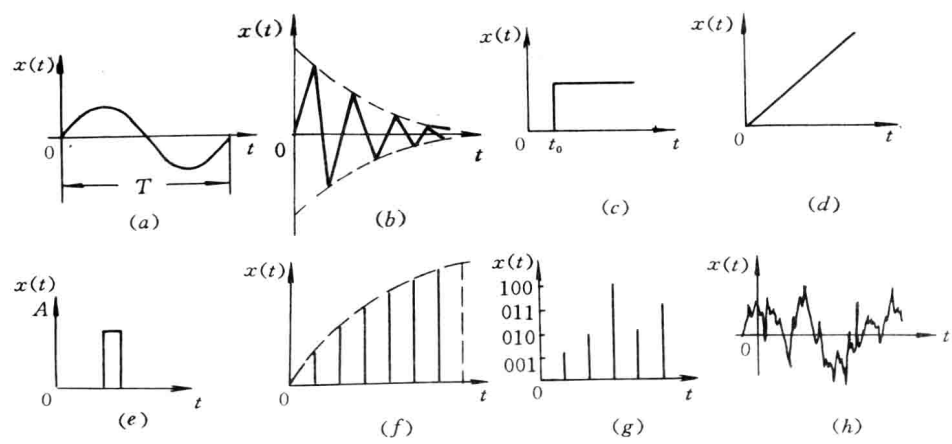
图 1-1 各种信号波形图
