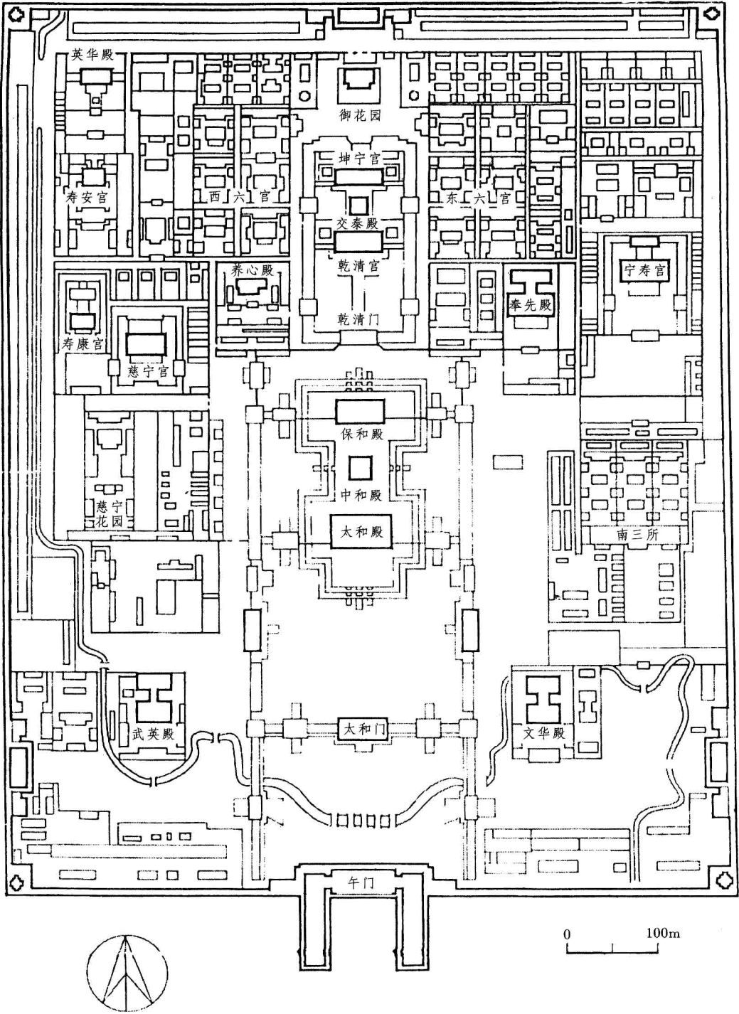
图三 清代紫禁城总平面图（乾隆初年）
