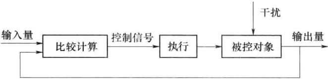
图 1.3.9 按偏差调节控制方框图
