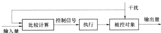
图 1.3.8 按干扰补偿控制方框图
