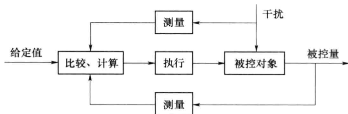
图 1.3.6 水池水位人工控制系统的方框图
