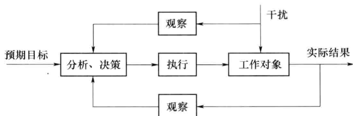
图 1.3.5 水池水位人工控制系统的职能图
