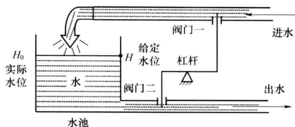
图 1.3.3 水池水位阀门联动控制系统示意图
