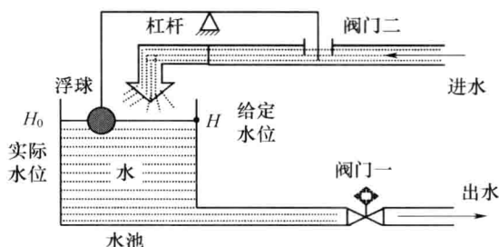
图 1.3.4 水池水位浮球控制系统示意图
