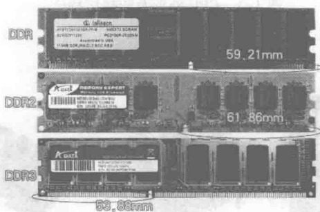
(f) DDR、DDR2、DDR3 内存对比
