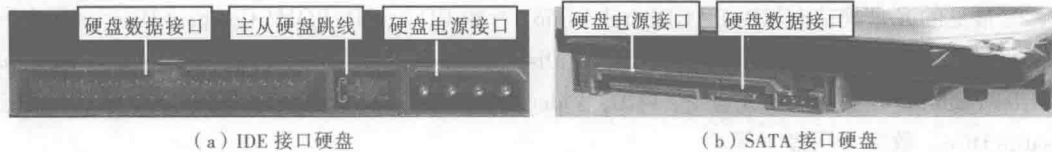
图 1-7 硬盘背部接口
