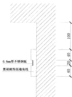
墙角线大样图
