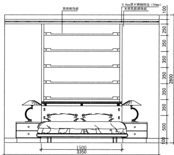
N二层主卧背景墙立面图
