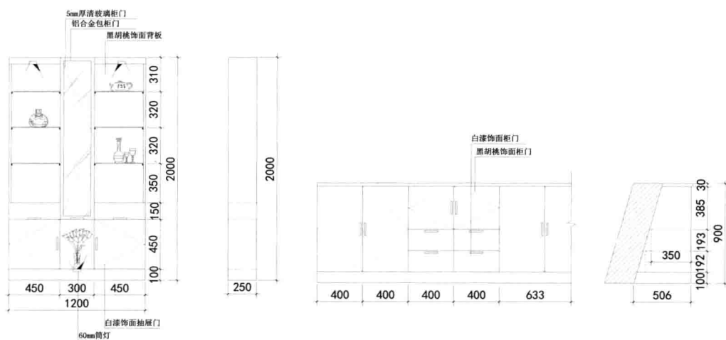
P起居室茶柜立面图
