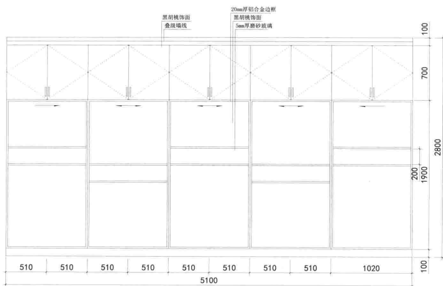
K储藏室立面图
