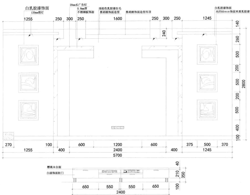
A客厅背景墙电视柜立面图
