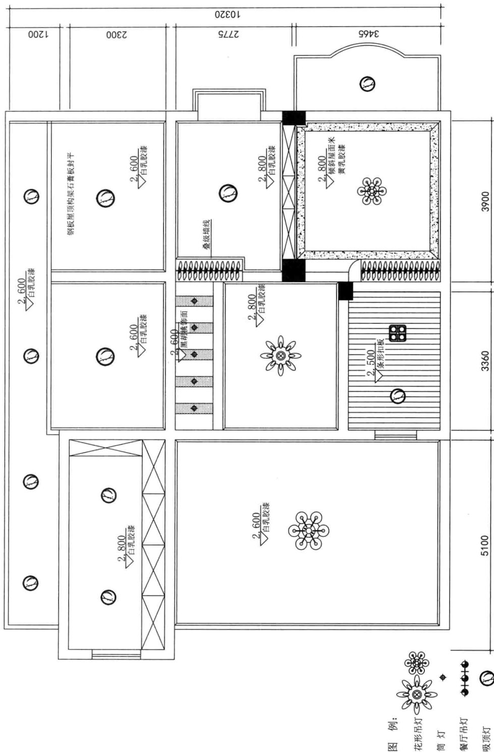
二层顶面布置图
