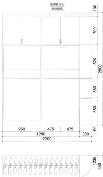
L二层主卧衣柜立面图
