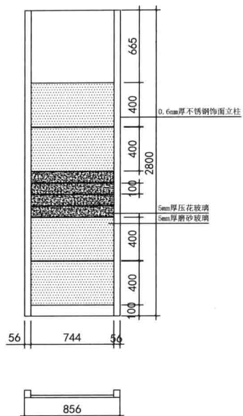
I主卧套房玄关立面图
