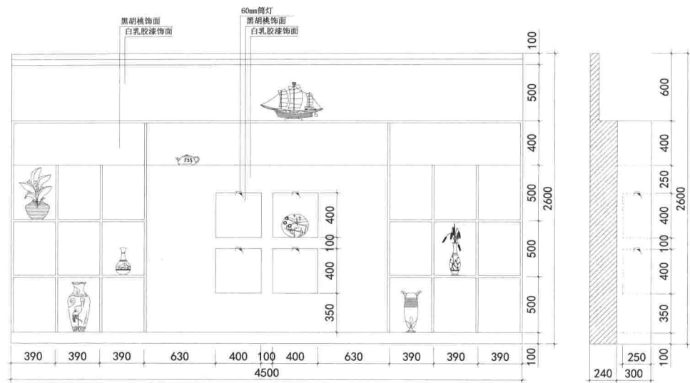
R平台书房综合柜立面图
