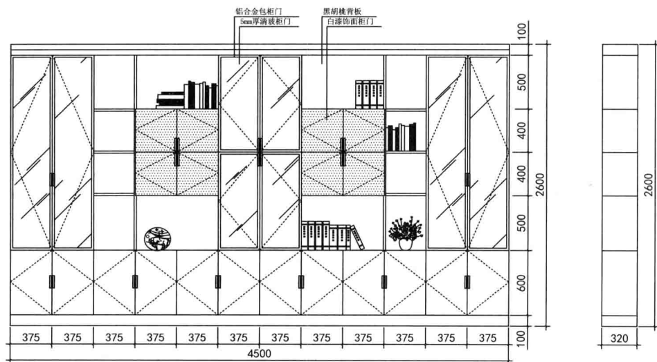
S平台书房书柜立面图
