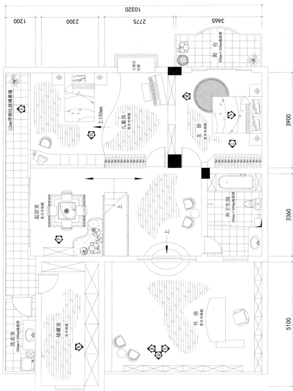
二层平面布置图
