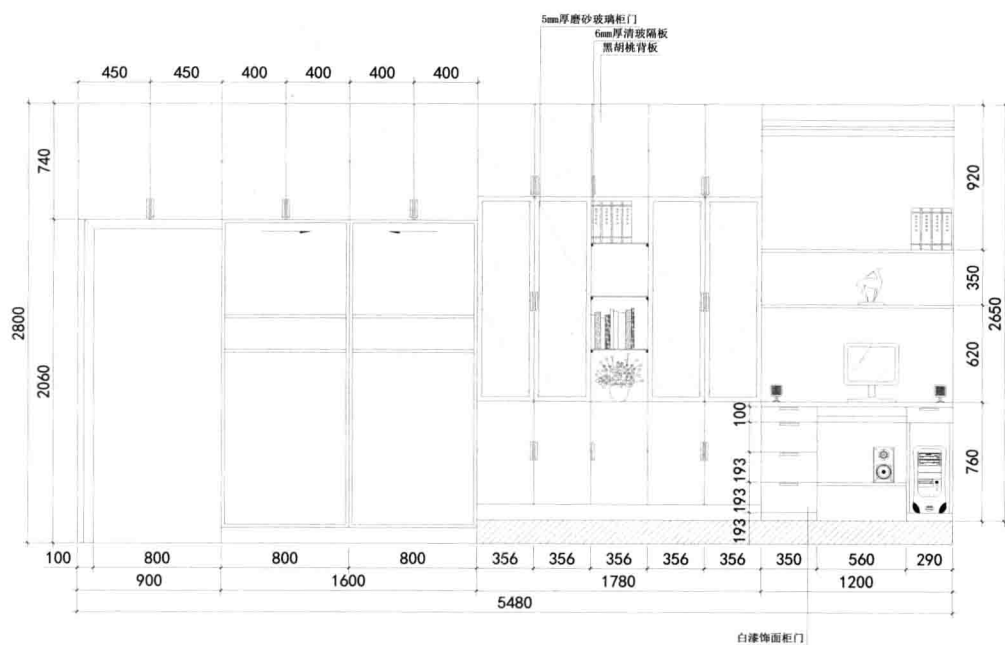
0儿童房衣柜书桌柜立面图
