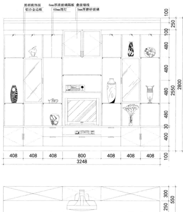
M二层主卧博物电视柜立面图
