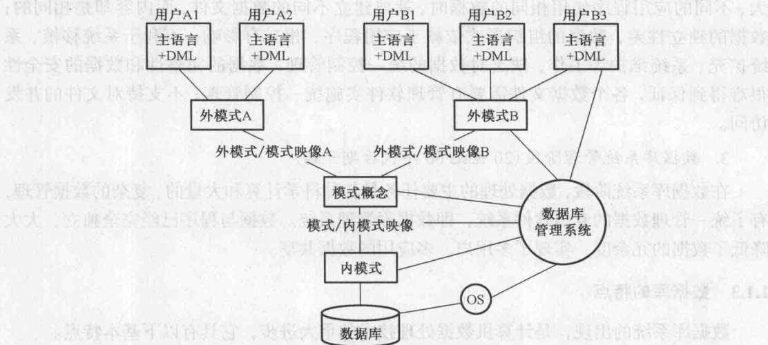
图 1-1 数据库系统的体系结构
