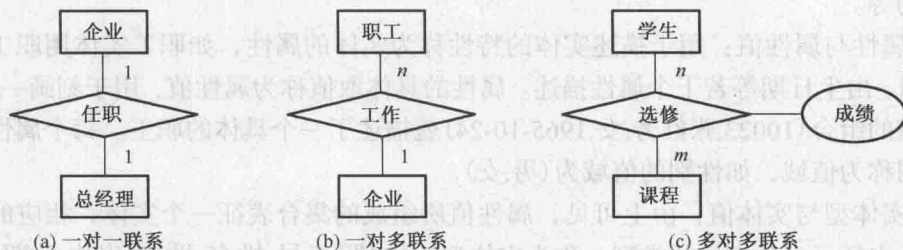
图 1-3 简单 E-R 方法表示
