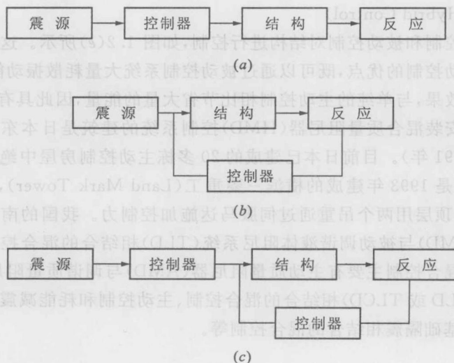
图 1.3 主动控制形式或类型
