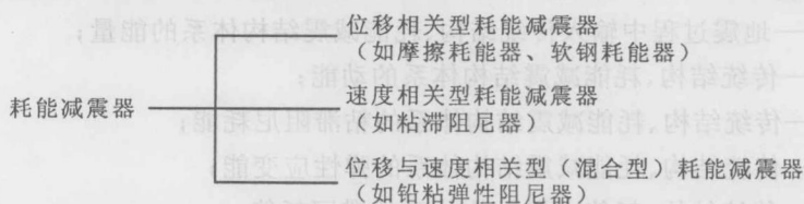
图 1.5 耗能减震器按与位移和速度的相关性分类
