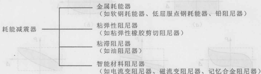
图 1.6 耗能减震器按耗能材料分类
