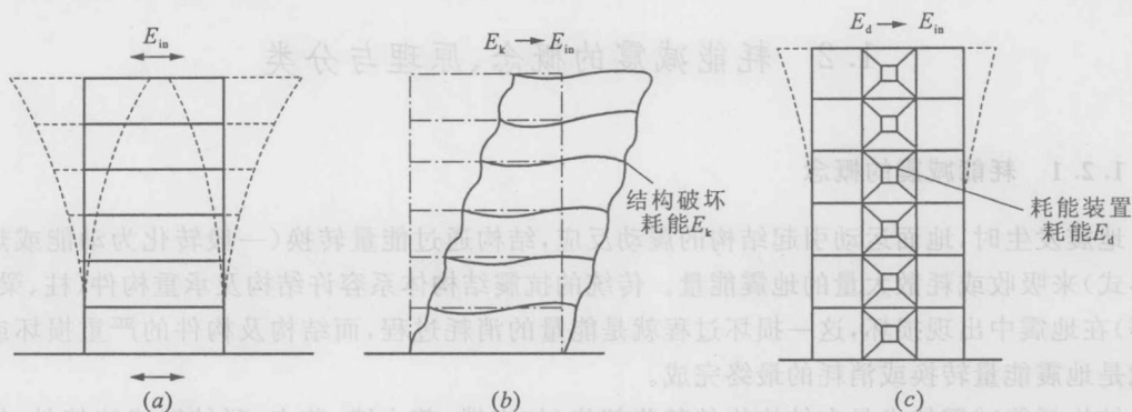
图 1.4 结构能量转换途径对比
