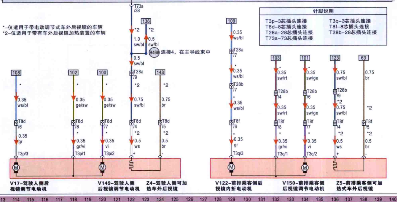
J519-车载电网控制单元
