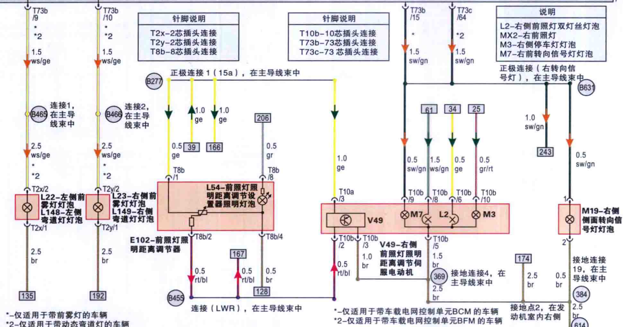
J519-车载电网控制单元
