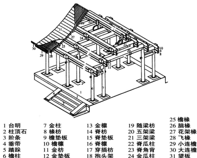
古建筑“墙倒屋不倒”的构架形式
