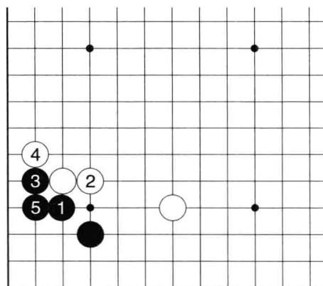
3图 消极
