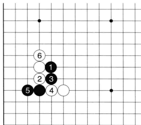
3图 黑无理
