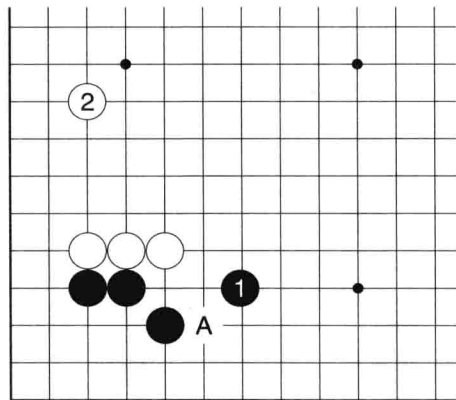
3图 弱点
