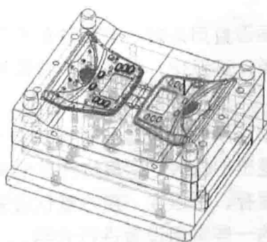
图 1-4 电子设备外壳模具机构
