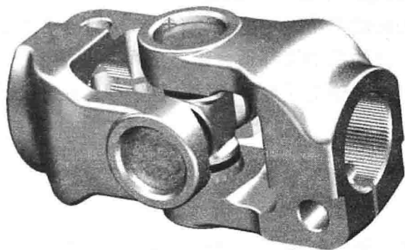
图 1-1 万向联轴器实体
