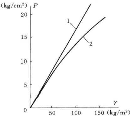
图 1-2 \text{SF}_6 压力变化 ( t=20^{\circ}\text{C} )
