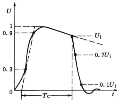
图 1-6 截波标准波 T_c —截断时间； U_i —截断时刻电压
