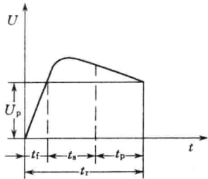
图 1-7 放电时间的各组成部分
