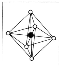
图 1-1 SF 6 分子结构 ○—F 原子；●—S 原子
