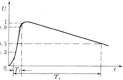
图 1-5 标准雷电冲击电压波形 T_{fi} —波头长度； T_t —波长时间
