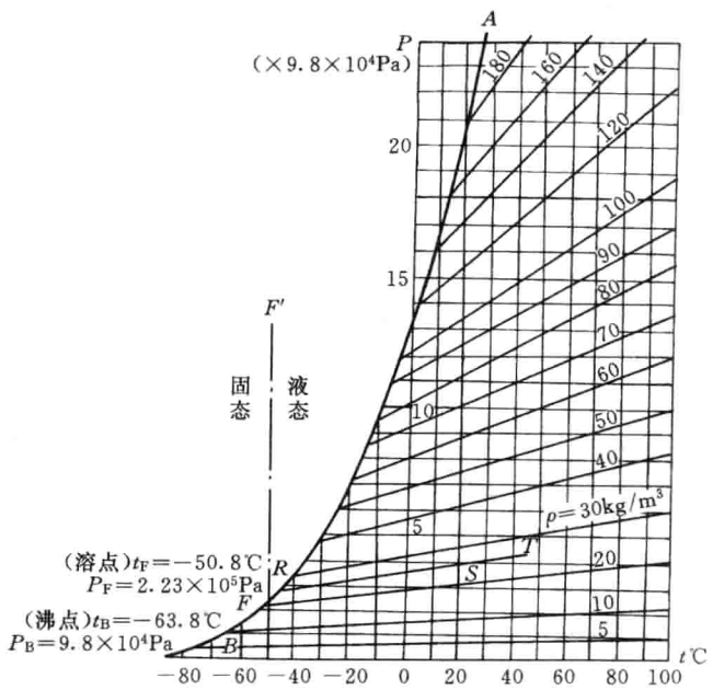
图 1-3 SF_6 的状态参数
