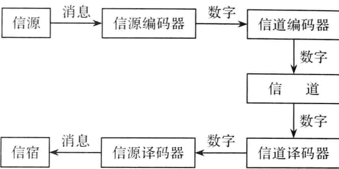
图 1.1 基本的通信系统模型
