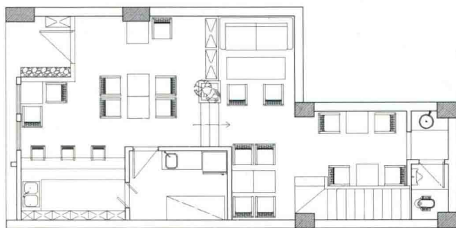
一楼平面布置图
