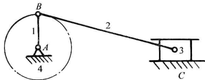
图 2-13 平面连杆机构
