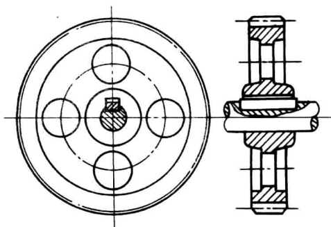
图 1-2 齿轮
