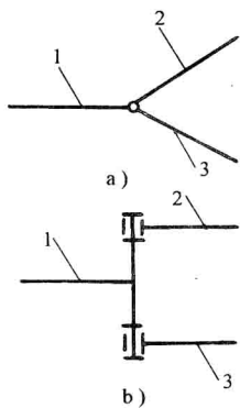
图 2-17 复合铰链
