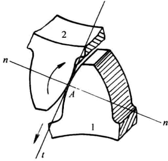
图 2-2 高副
