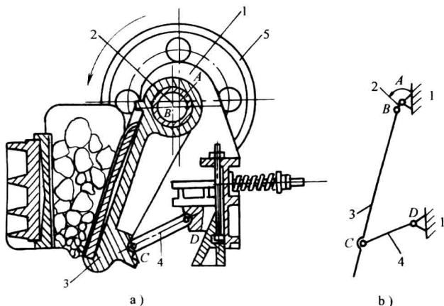
图 2-10 颚式破碎机及其机构运动简图 1—机架 2—偏心轴 3—动颚 4—肋板 5—轮
