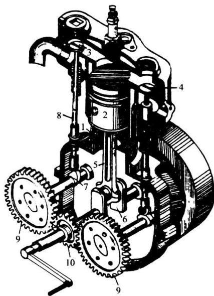
图 1-1 内燃机
