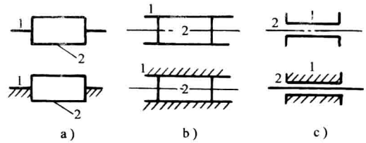
图 2-5 移动副的表示方法
