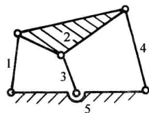
图 2-16 F=0 的构件组合
