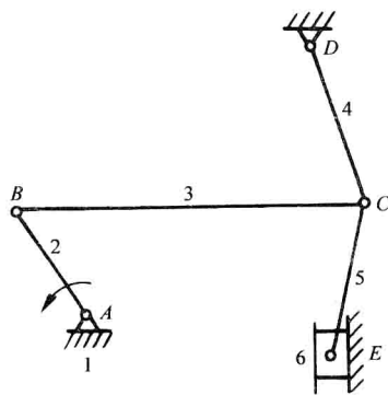
图 2-18 带复合铰链机构
