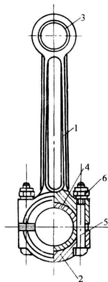
图 2-1 内燃机连杆
