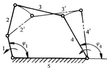
图 2-14 原动件数 < F
