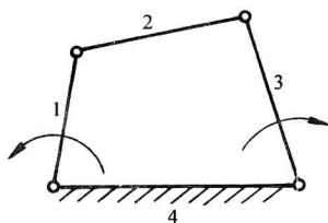
图 2-15 原动件数 > F
