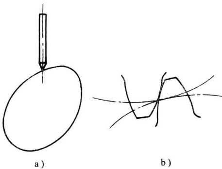
图 2-6 高副的表示方法
