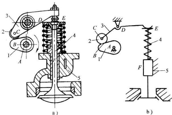
图 2-9 发动机配气机构
