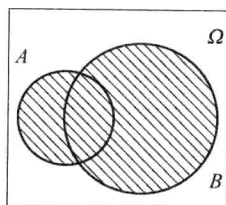
图 1.2 A \cup B
