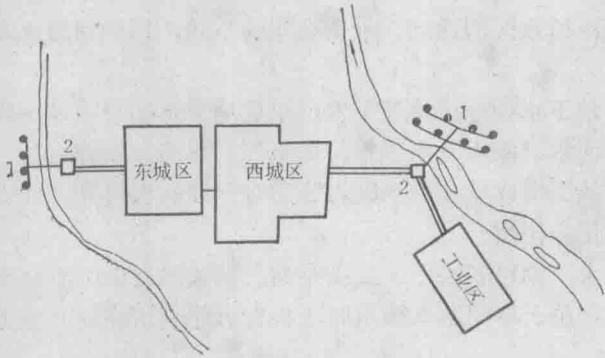
图 1-6 分地区给水系统 1—管井群; 2—泵站
