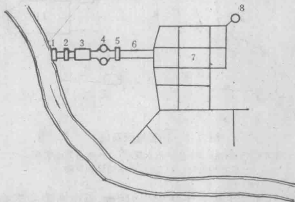
图 1-1 给水系统示意
