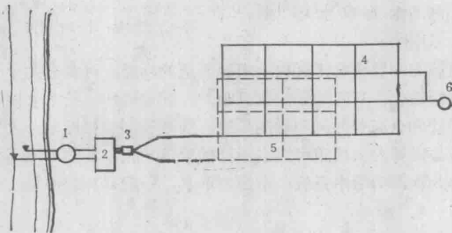
图 1-4 分压给水系统
