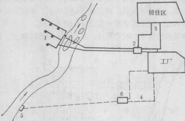
图 1-3 分质给水系统
