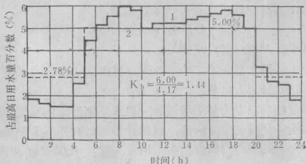
图 2-1 城镇用水量变化曲线
