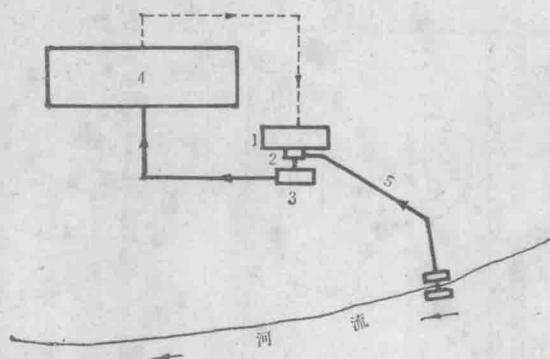
图 1-8 循环给水系统
