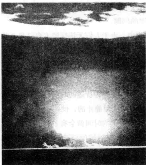
□ 原子弹爆炸 摄影
