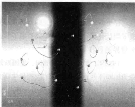
□ 黑洞 合成图片
