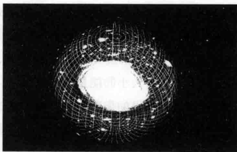
□ 宇宙的终结 合成图片
