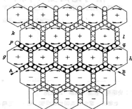
□ 以太合成 示意图
