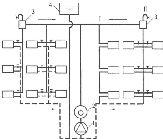
图 1.8 机械循环上供下回式热水供暖系统
