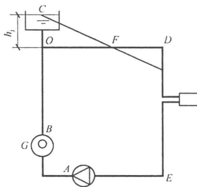
图 1.7 机械循环系统膨胀水箱与系统的错误接法
