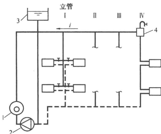
图 1.15 异程式系统
