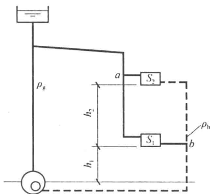
图 1.3 自然循环双管上供下回式系统
