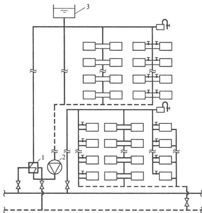
图 1.17 设热交换器的分区式热水供暖系统
