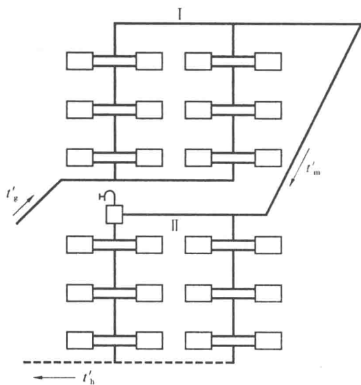
图 1.12 机械循环混合式热水供暖系统
