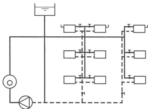
图 1.10 机械循环中供式热水供暖系统
