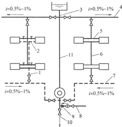
图 1.2 自然循环热水供暖系统
