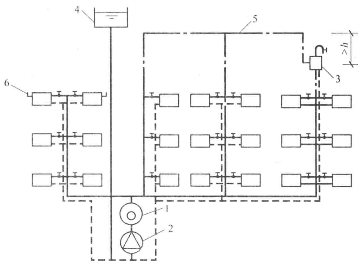
图 1.9 机械循环双管下供下回式热水供暖系统
