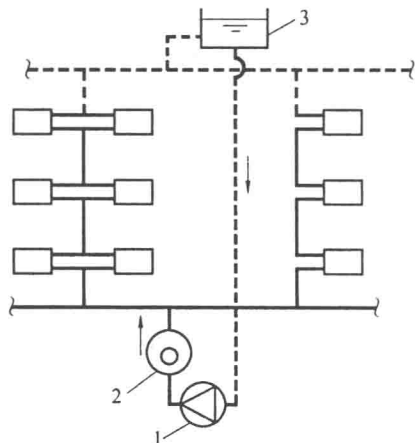
图 1.11 机械循环下供上回(倒流)式热水供暖系统
