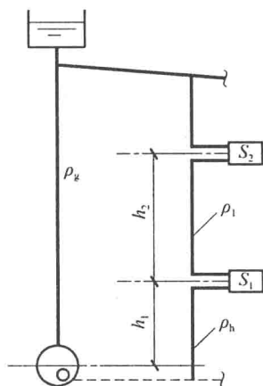
图 1.4 自然循环单管系统上供下回式
