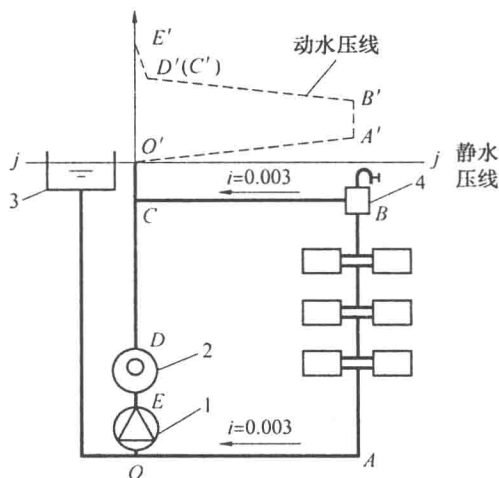
图 1.6 机械循环热水供暖系统
