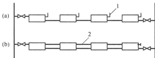
图 1.13 水平单管顺流式系统
