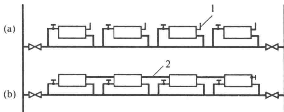
图 1.14 水平单管跨越式系统
