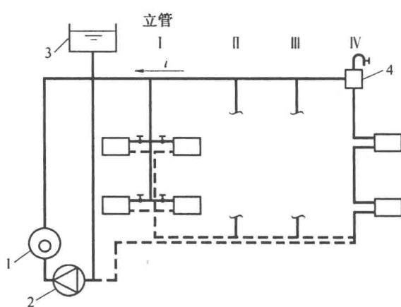
图 1.16 同程式系统
