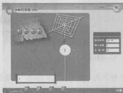
图 5 打字游戏
