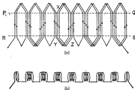
图 10 圆筒型电动机绕组端部的优点
