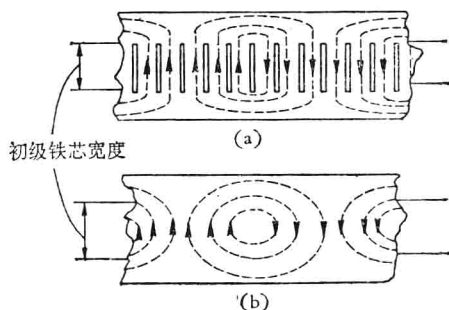
图 5 开槽式次级片图(a)和片状转子图(b)中的电流分布
