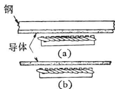
图7 两种单边型直线电动机
