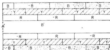
图 11 圆筒型电动机的三层连续结构
