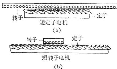
图 3 直线电动机的两种基本类型
