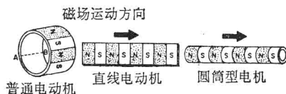
图 9 圆筒型电动机的由来
