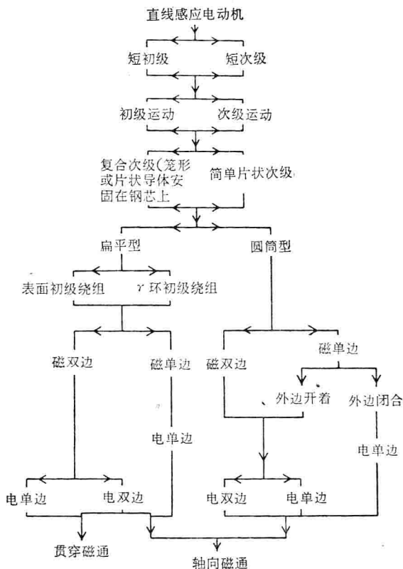
图 12 直线感应电动机的拓扑分类
