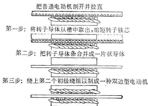
图 4 “片状转子”电动机的发展过程
