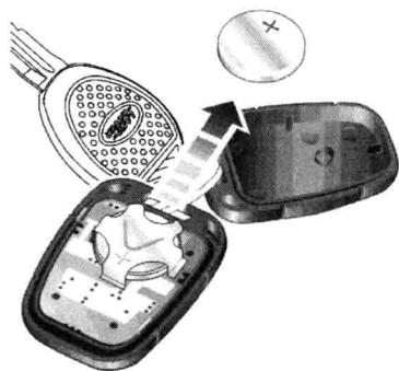
图 1-1-1 遥控器电池更换
