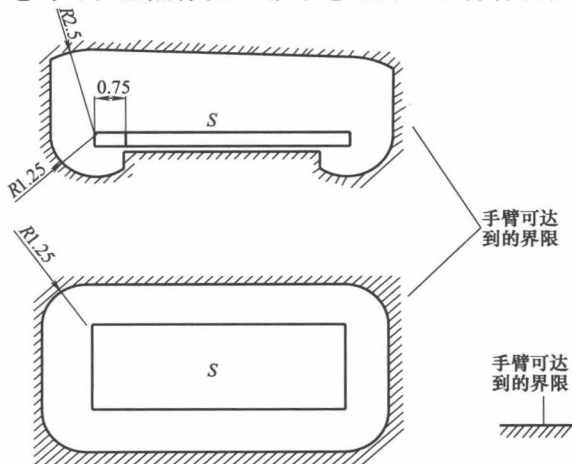
图 B.1 伸臂范围
