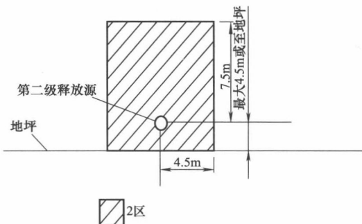
图2.3.7 易燃物质轻于空气、通风良好的生产装置区
