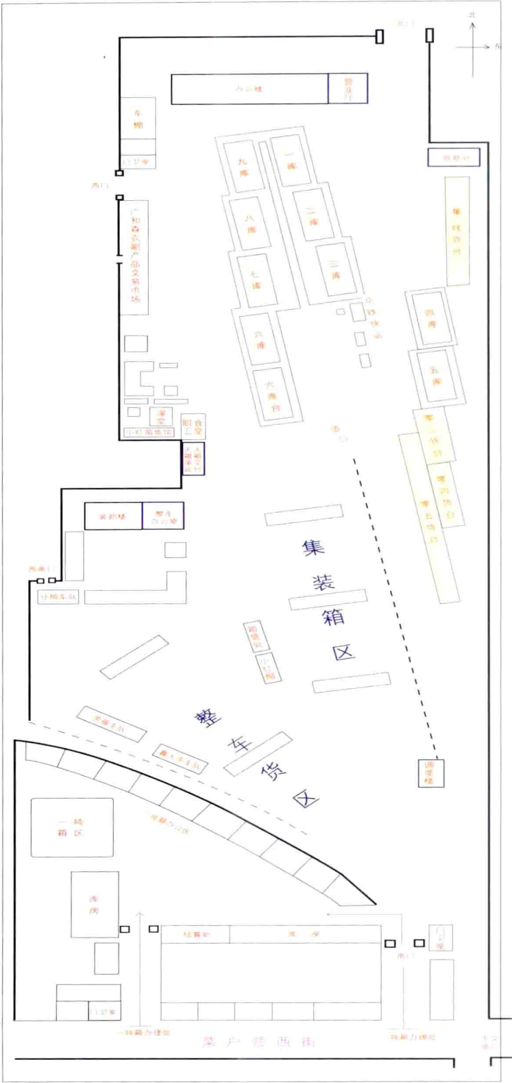
广安门站站场平面图
