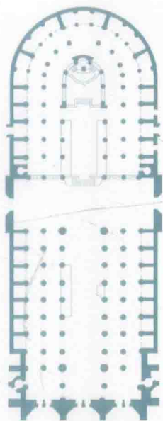
平面图
