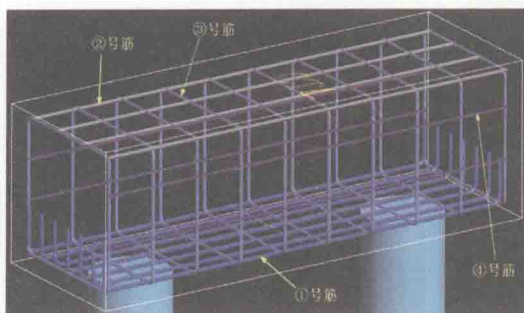
图1 承台三维钢筋
