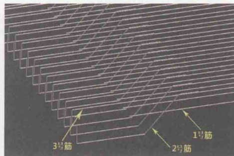
图2 防水底板三维钢筋
