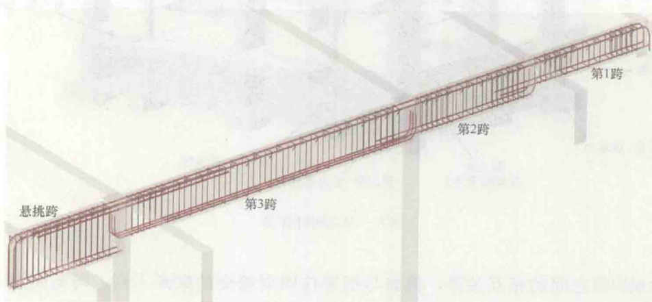
图6 梁三维钢筋
