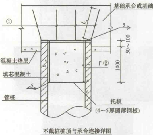
图 1-1-1 桩与承台的连接
