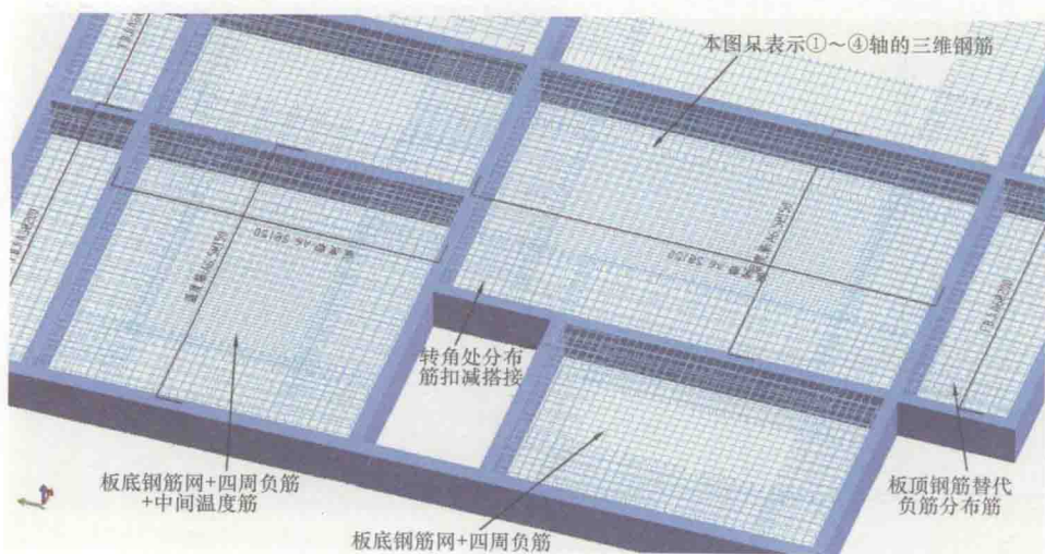
图7 现浇板三维钢筋
