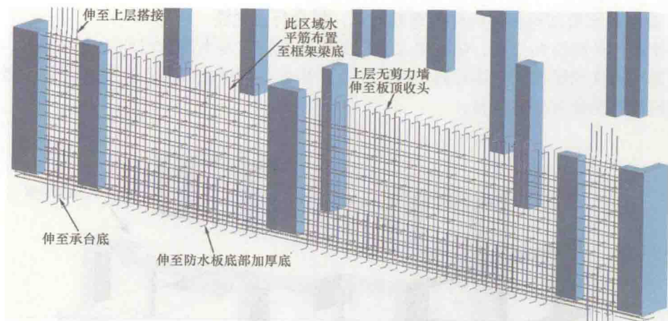
图5 剪力墙三维钢筋
