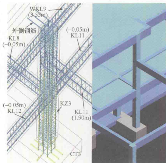
图3 框架柱三维钢筋
