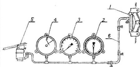
1 压力源 2 灵敏表 3 指示表 4 压力表 5 手压泵 6 连接导管
