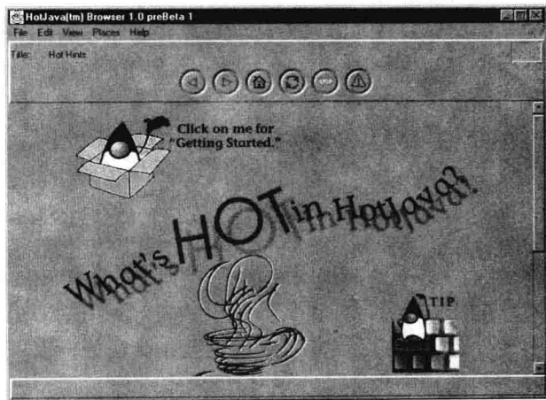
图 2 HotJava 浏览器
