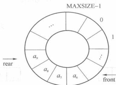
图 1-6 循环队列
