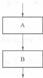
图 1-11 顺序结构
