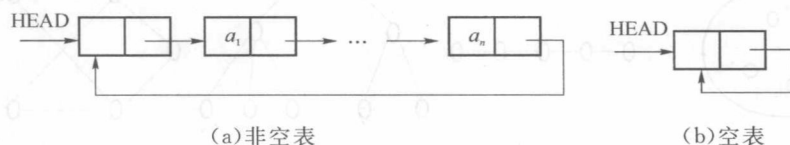
图 1-2 带头结点的单循环链表
