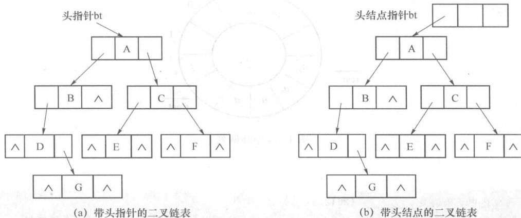
图 1-9 二叉树的二叉链表表示
