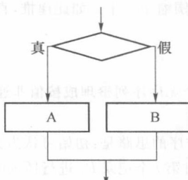
图 1-12 选择结构
