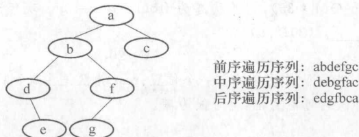
图 1-10 二叉树的遍历序列
