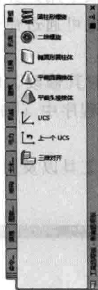
图 1-15 工具选项板
