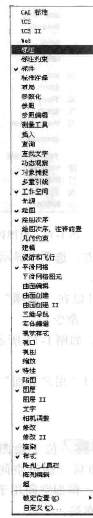
图 1-8 “工具” 菜单
