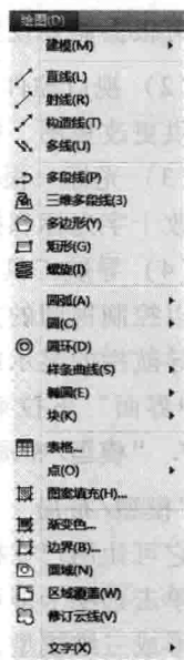
图 1-10 “绘图” 菜单
