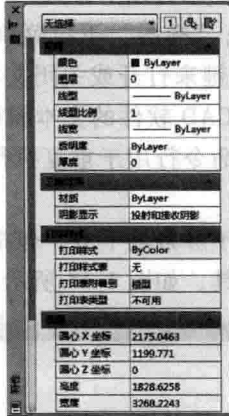
图 1-16 特性选项板
