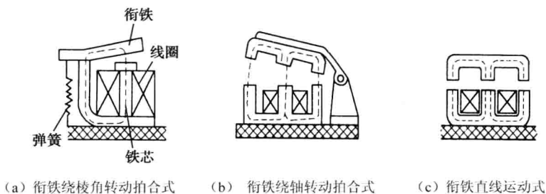
图 1.1 常用的电磁机构的结构
