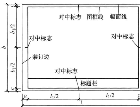
图 1-2 A0 ~ A3 横式幅面 (二)
