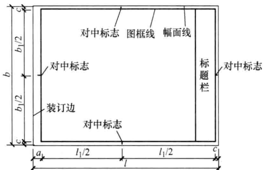
图 1-1 A0 ~ A3 横式幅面 (一)
