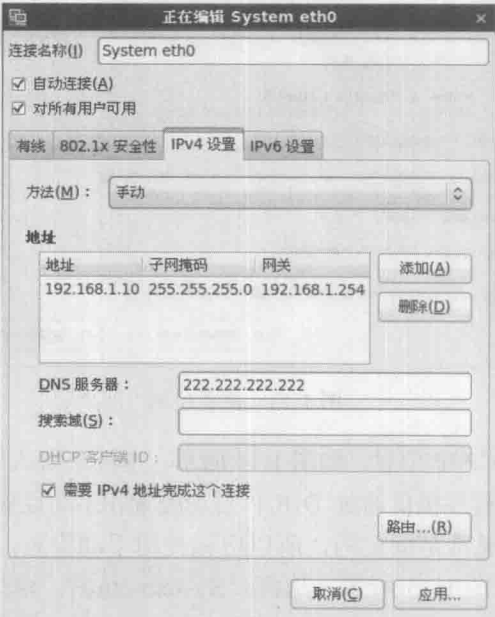
图 1-16 编辑接口 eth0
