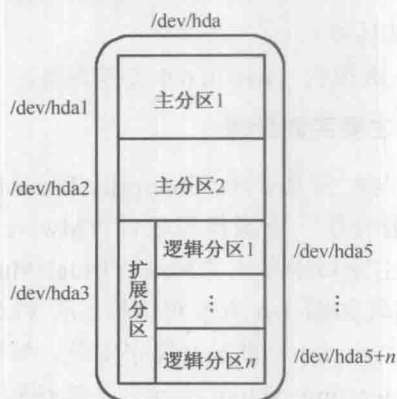
图 1-5 扩展分区和逻辑分区表示法
