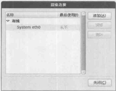
图 1-15 网络连接
