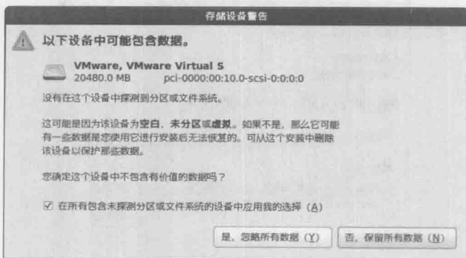
图 1-13 磁盘检测
