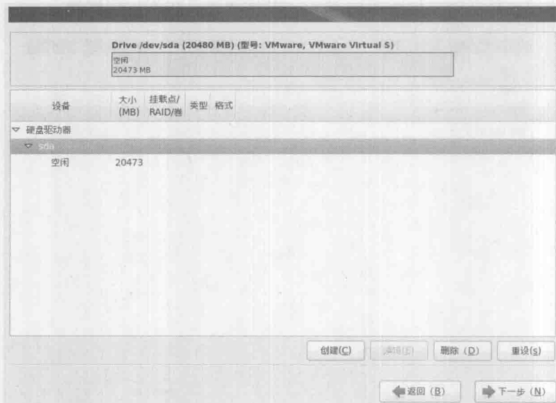
图 1-20 磁盘分区
