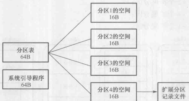
图 1-3 扩展分区
