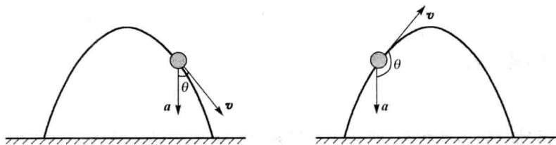
图 1-7 抛体运动
