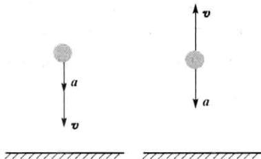
图 1-5 直线运动
