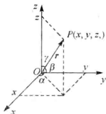
图 1-2 位置矢量
