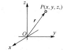
图 1-1 直角坐标系
