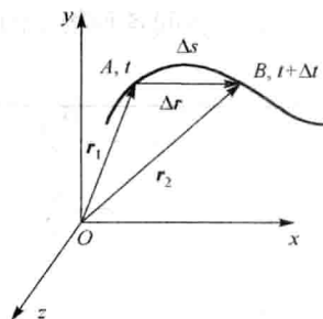
图 1-3 位移矢量
