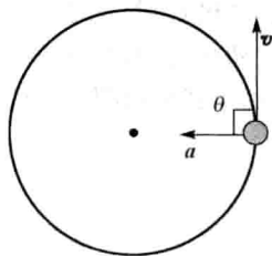
图 1-6 圆周运动
