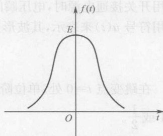
图 1-9 高斯函数
