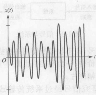
图 1-2 随机信号
