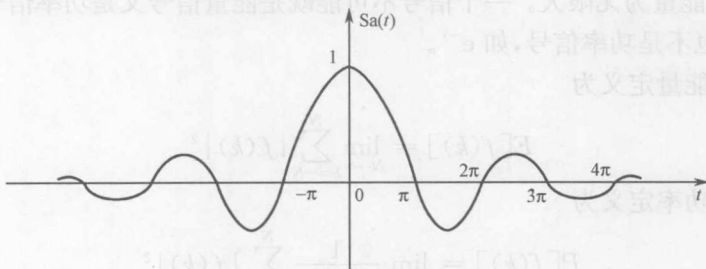
图 1-8 抽样函数
