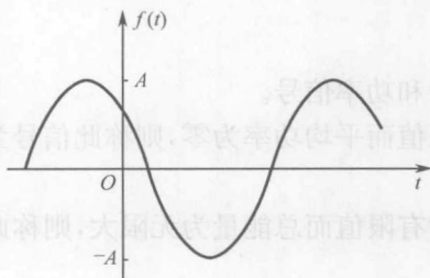
图 1-6 正弦函数
