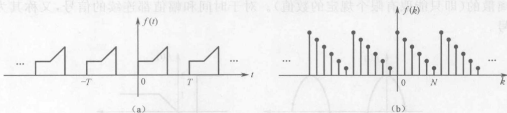
图 1-5 周期信号
