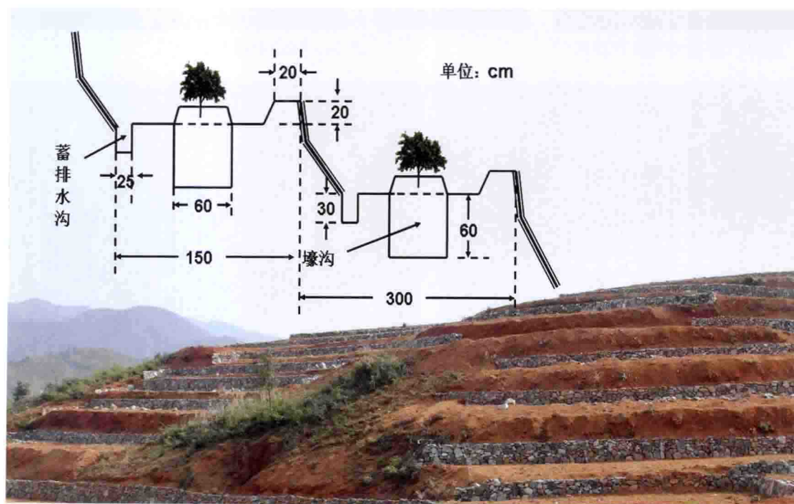
图27 带埂梯带状整地
