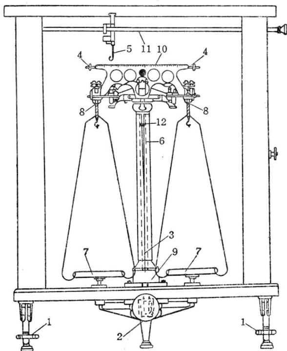
图Ⅱ—1 分析天平
