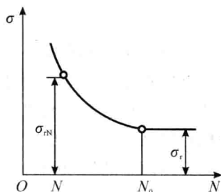
图 1-1 疲劳曲线
