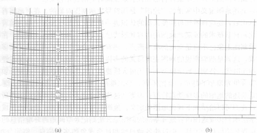
图 1.1 平面直角坐标系的构成 (a) 及其在地形图 (1:5 万) 上的表示 (b)
