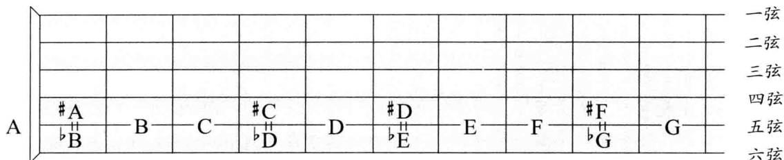
等音示意图
