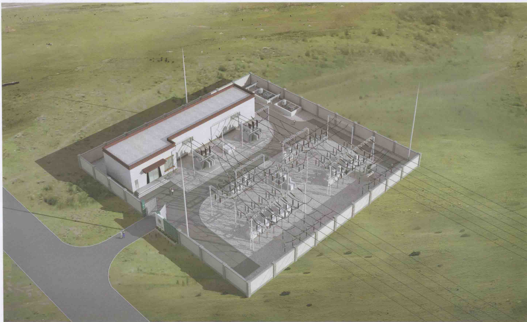
35kV变电站方案A—2鸟瞰效果图
