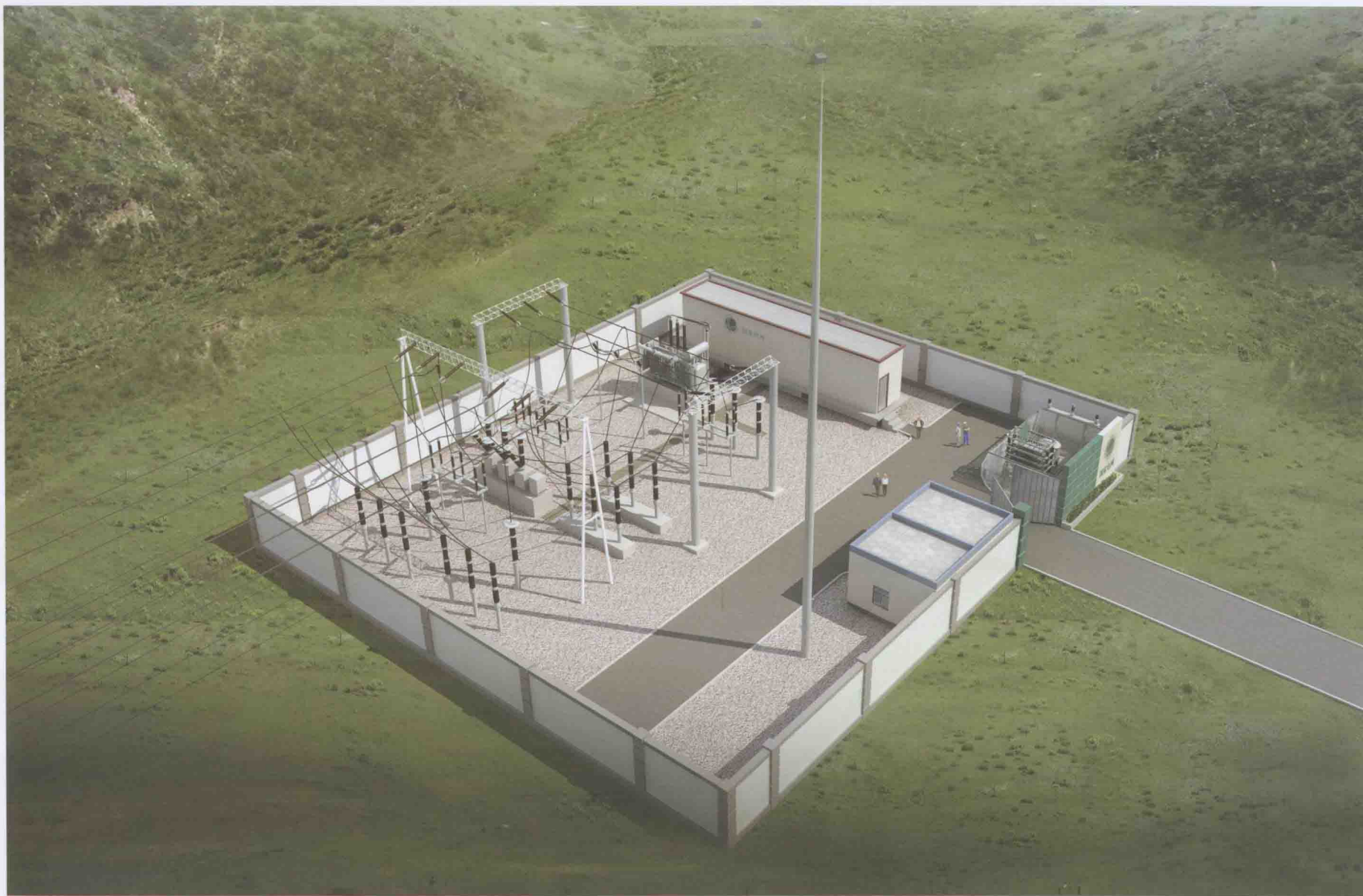
35kV变电站方案D—2方案鸟瞰效果图
