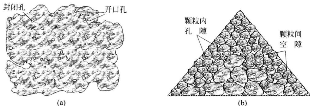
图 1-1 材料的孔隙与空隙结构示意图
