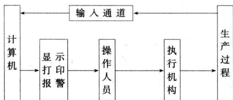
图 1-5 数据采集和操作指导控制结构
