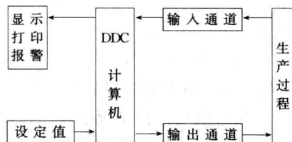
图 1-6 直接数字控制系统结构
