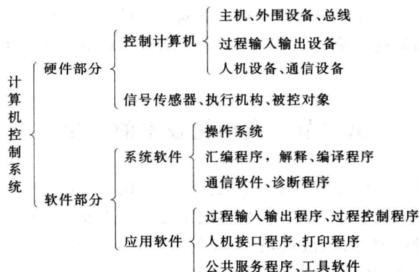
图 1-4 计算机控制系统的构成
