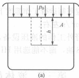
图 1-5 重力作用下静止的液体
