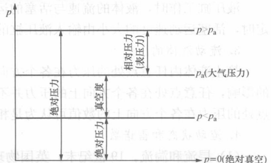
图 1-8 绝对压力、相对压力和真空度
