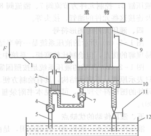
图 1-1 液压千斤顶工作原理图
