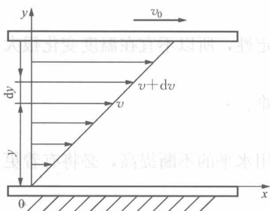
图 1-3 液体的黏性示意
