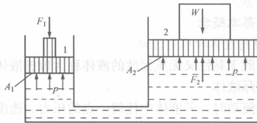
图 1-7 液压千斤顶的工作原理图
