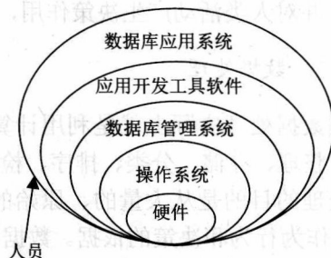
图 1-2 数据库管理系统在计算机中的地位
