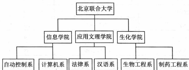
图 1-3 层次模型
