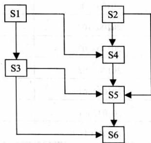
图 1-4 网状模型
