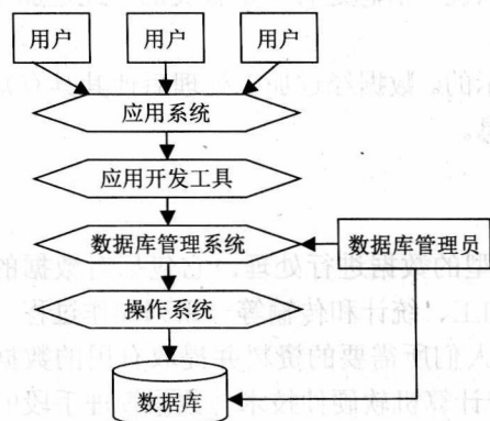
图 1-1 数据库系统的组成结构
