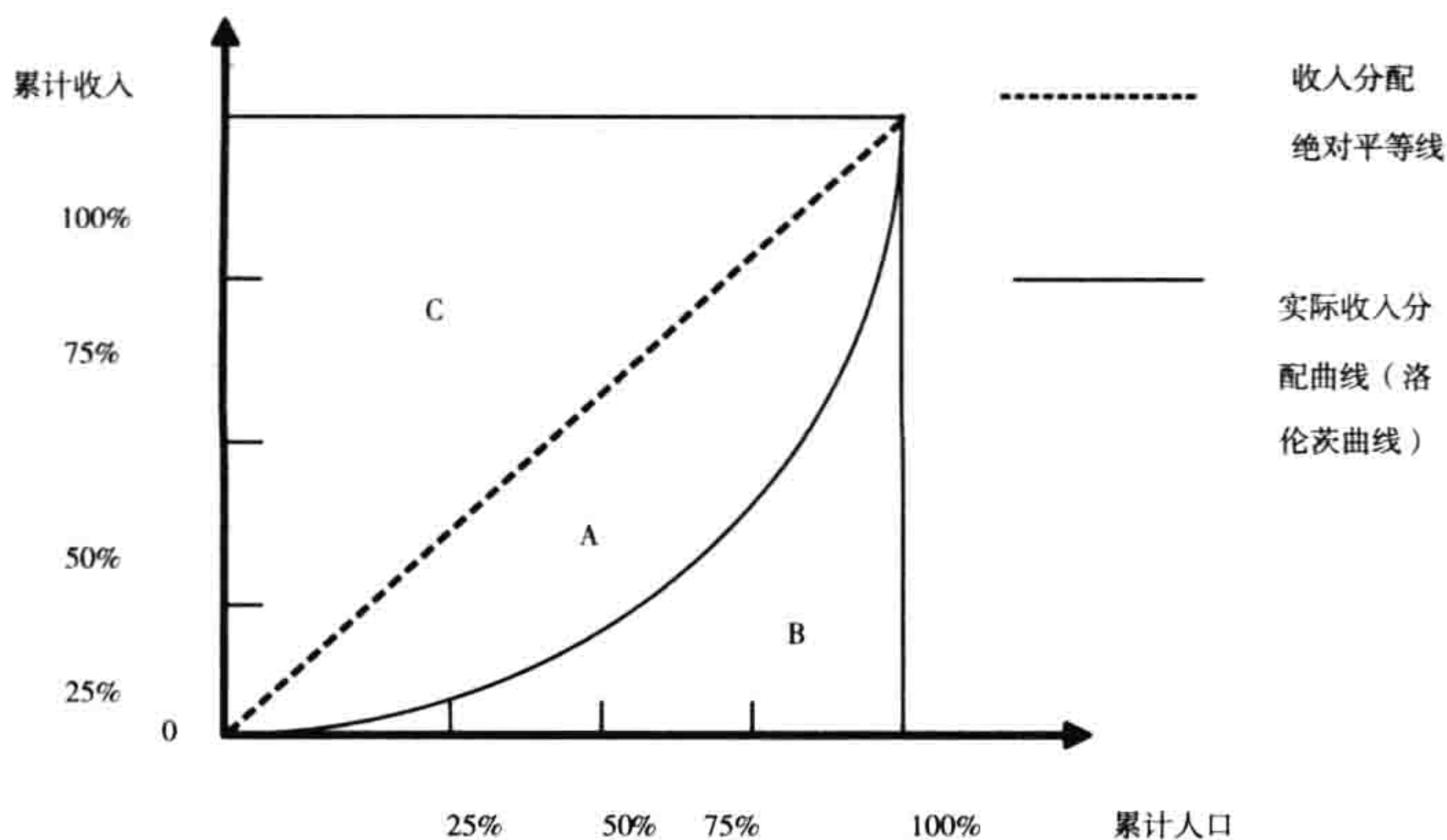
图 1-2 某国的洛伦茨曲线
