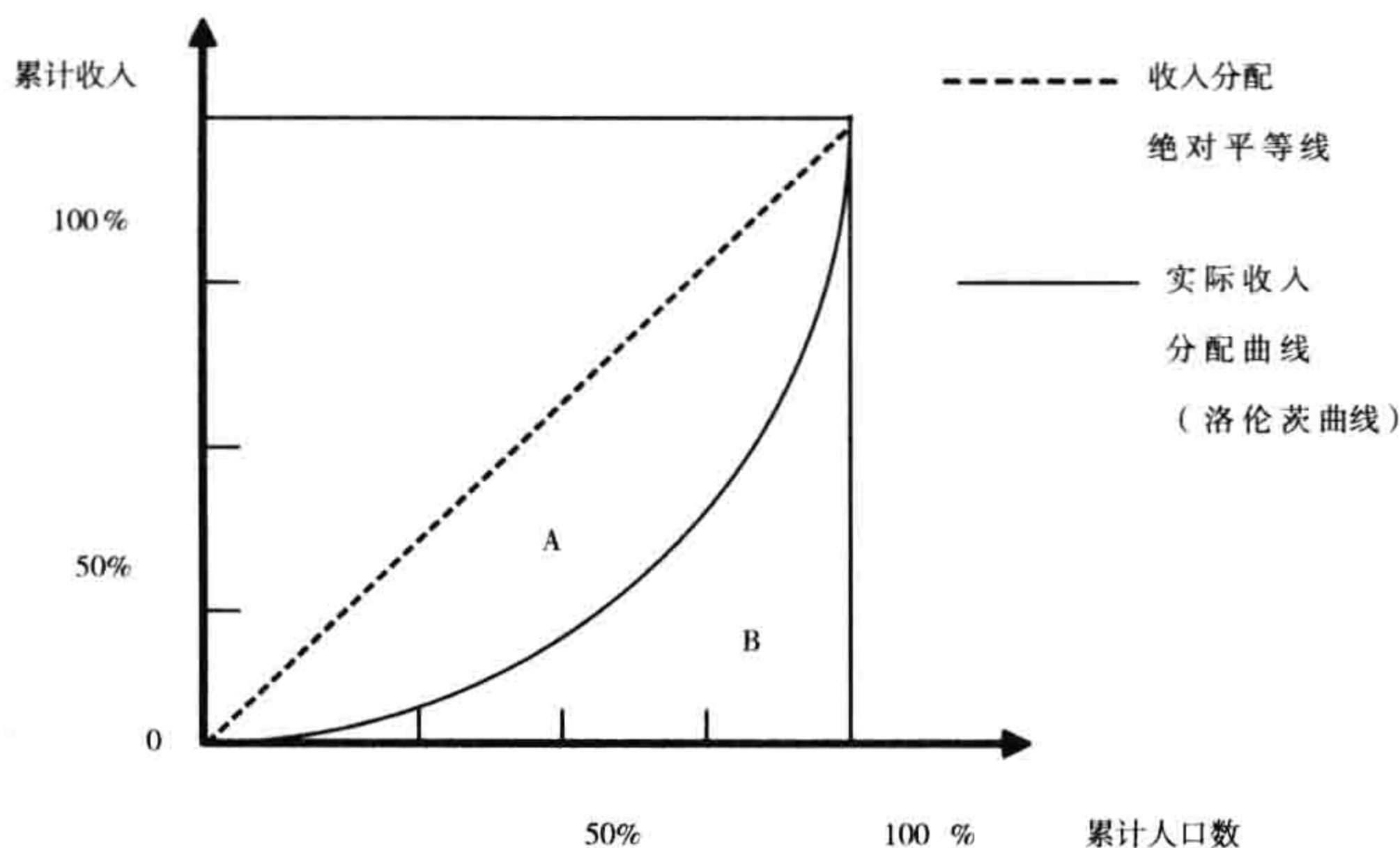
图 1-1 洛伦茨曲线
