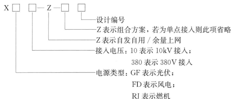
图 1-1 接入系统方案编号命名原则
