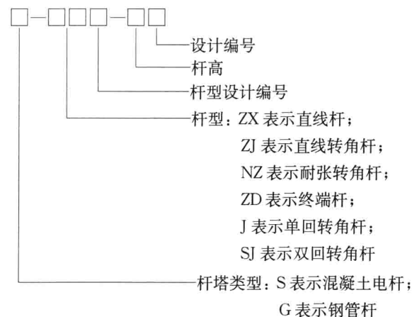
图 1-3 杆型编号命名原则
