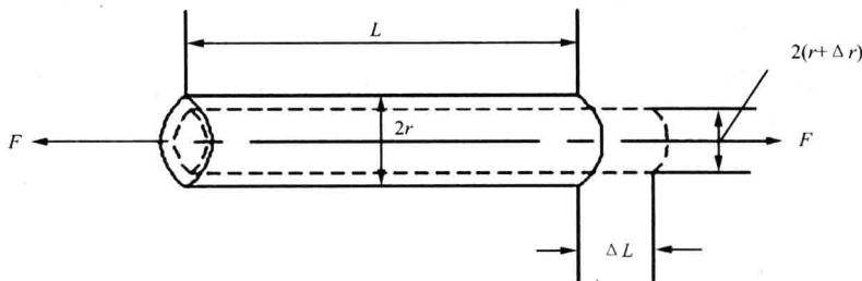
图 1-3 电阻丝拉伸应变示意图
