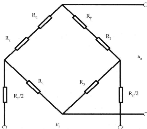
图 1-10 零漂移补偿电路
