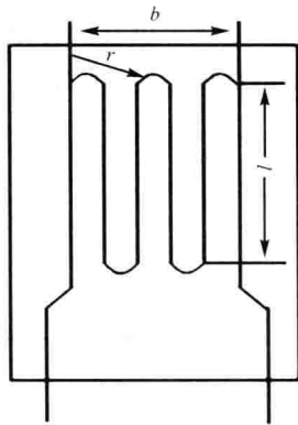
图 1-1 丝式应变片
