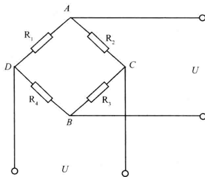
图 1-4 直流电桥
