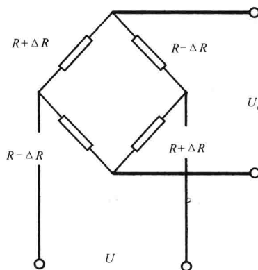
图 1-6 等臂电桥
