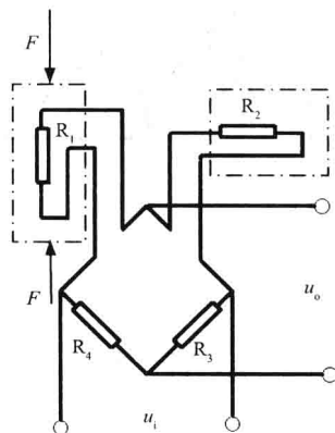
图 1-9 温度补偿电路
