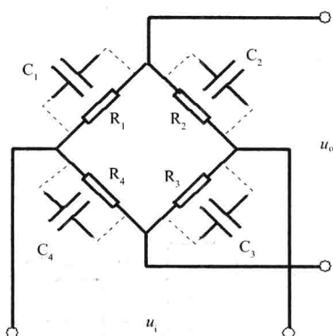
图 1-7 应变片等臂交流电桥
