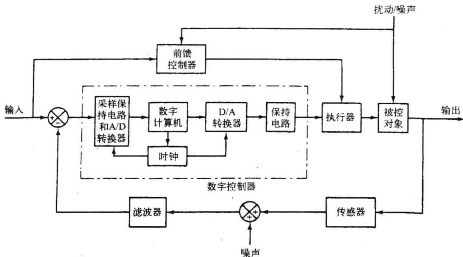
图 1-2 数字控制系统框图
