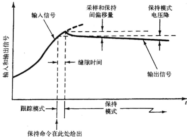
图 1-8 跟踪模式和保持模式
