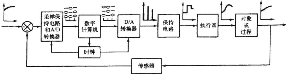
图 1-3 数字控制系统框图(图中信号以二进制或图形表示)
