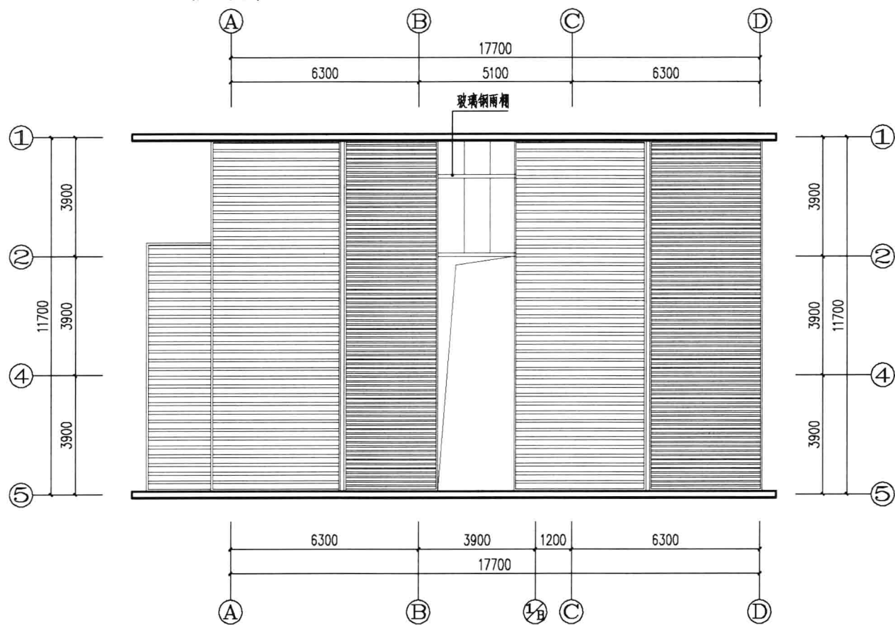
屋顶平面图
