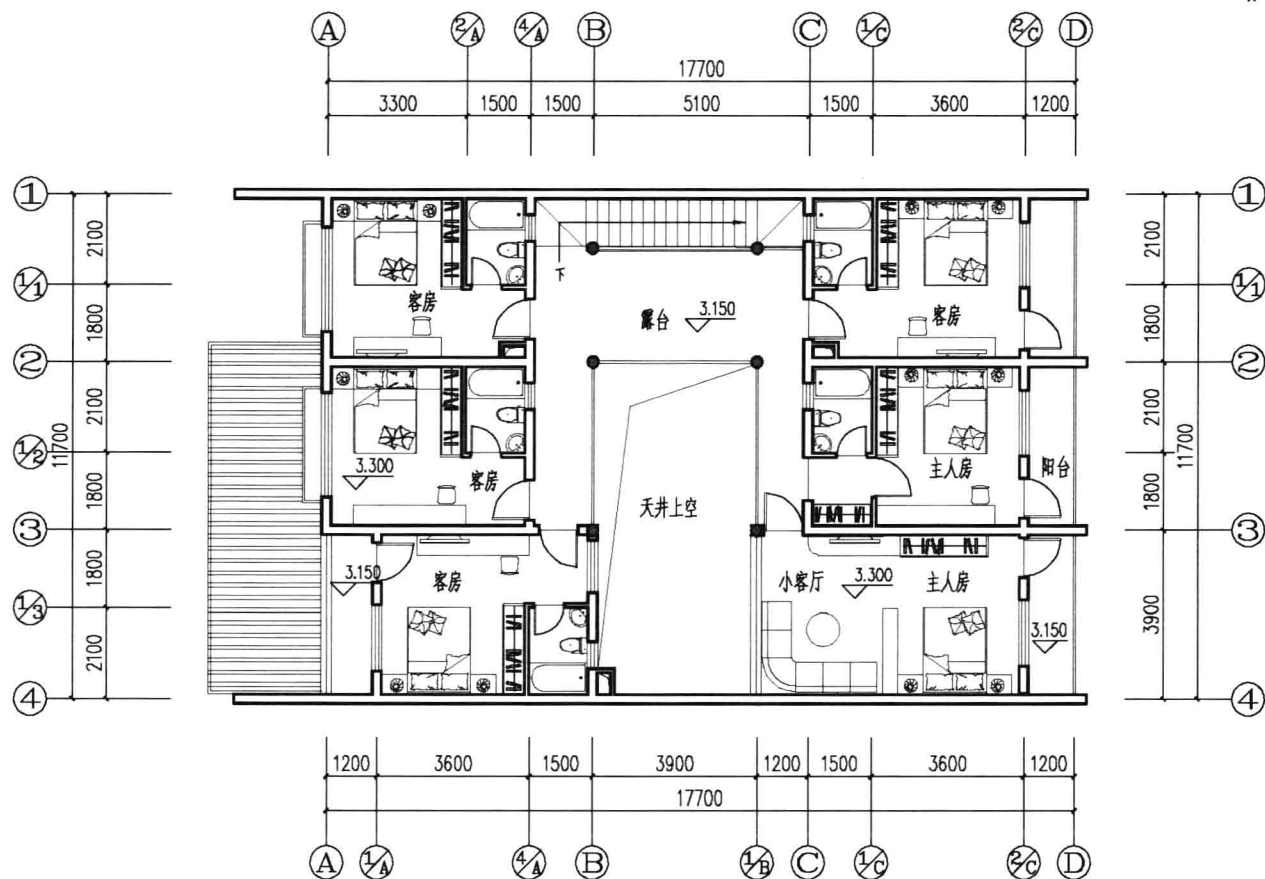
二层平面图
