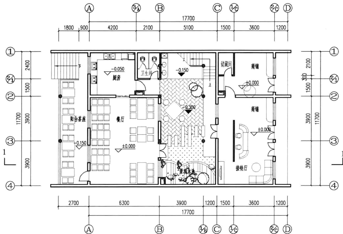
一层平面图
